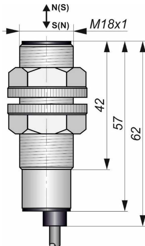
Габаритный чертеж
