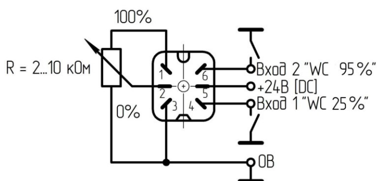
Схема подключения
