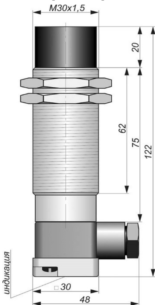
Габаритный чертеж
