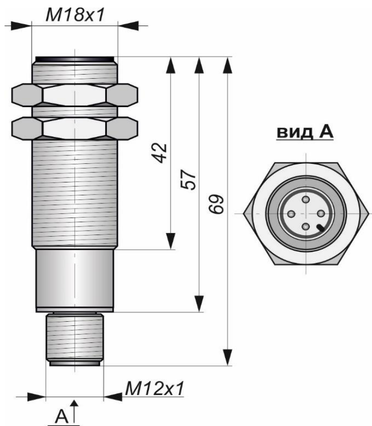
Габаритный чертеж
