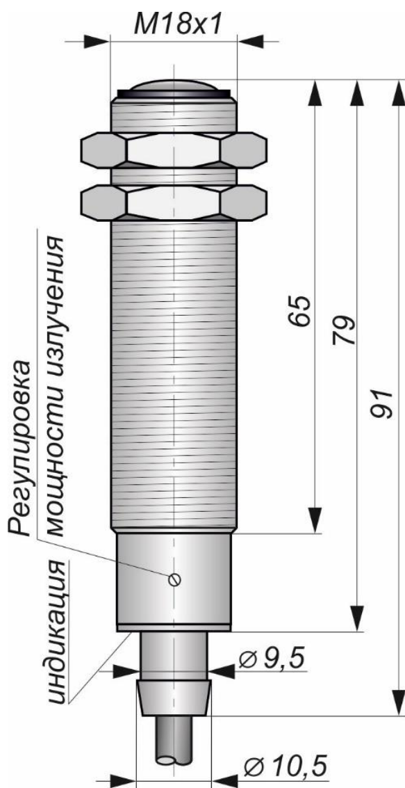
Габаритный чертеж
