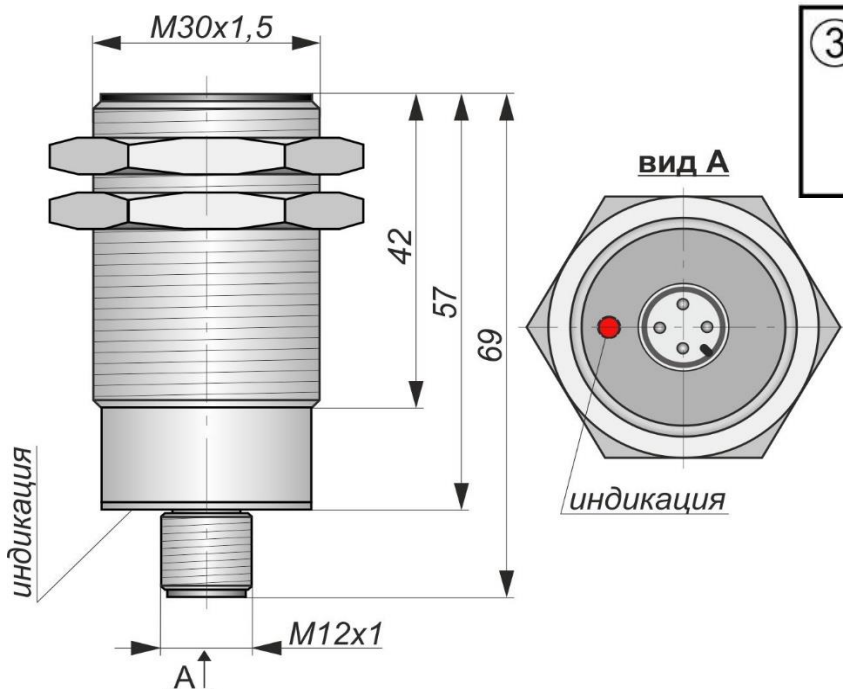
Габаритный чертеж
