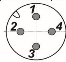
Цоколевка разъема
