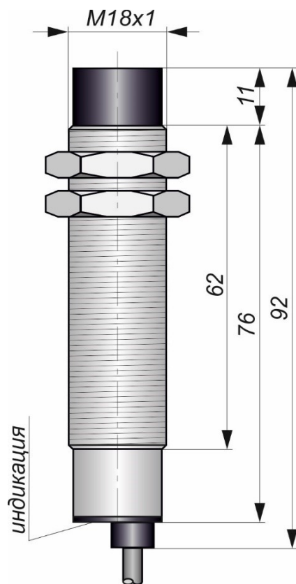
Габаритный чертеж
