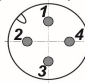
Цоколевка разъема
