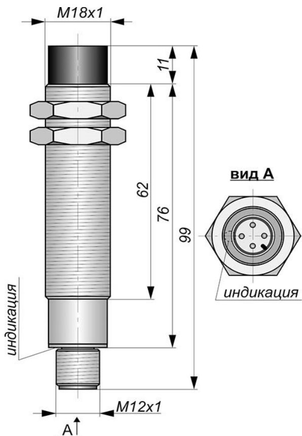
Габаритный чертеж
