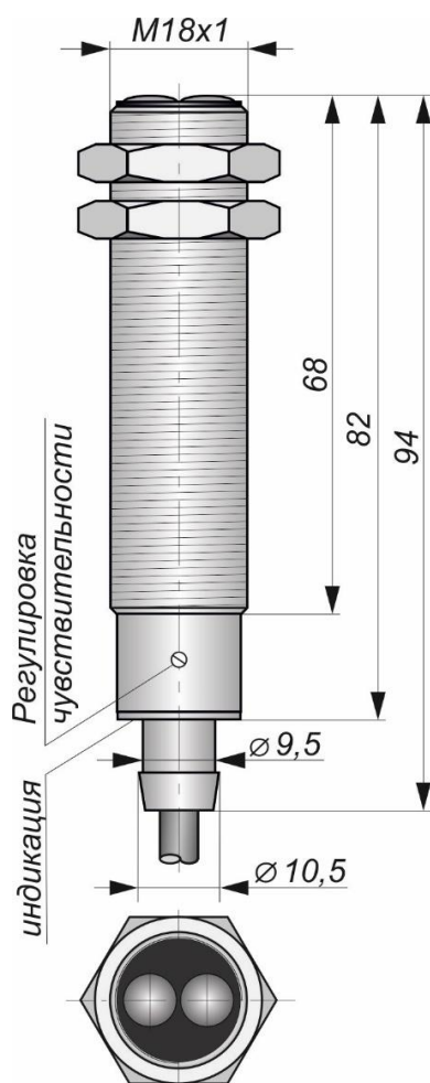
Габаритный чертеж
