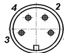
Цоколевка разъема
