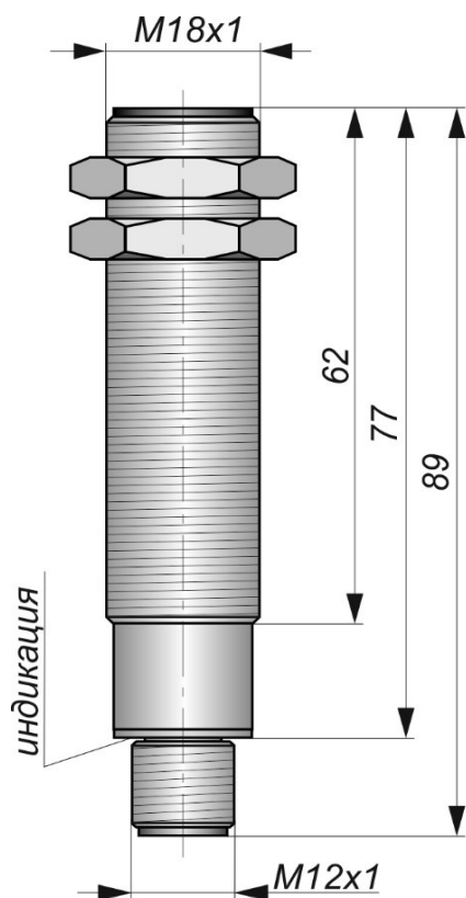
Габаритный чертеж
