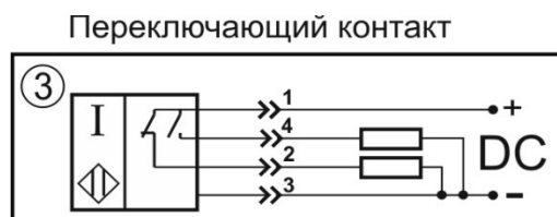
Схема соединения
