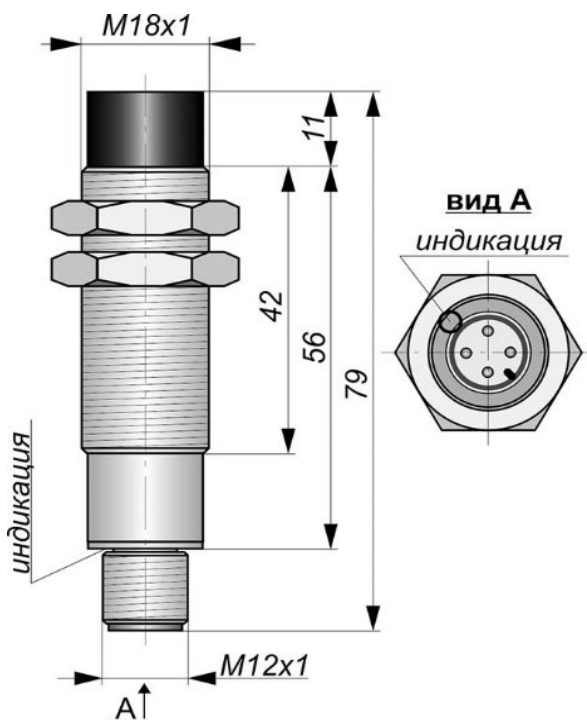
Габаритный чертеж
