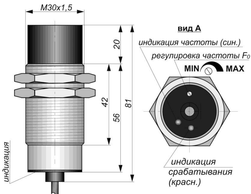
Габаритный чертеж
