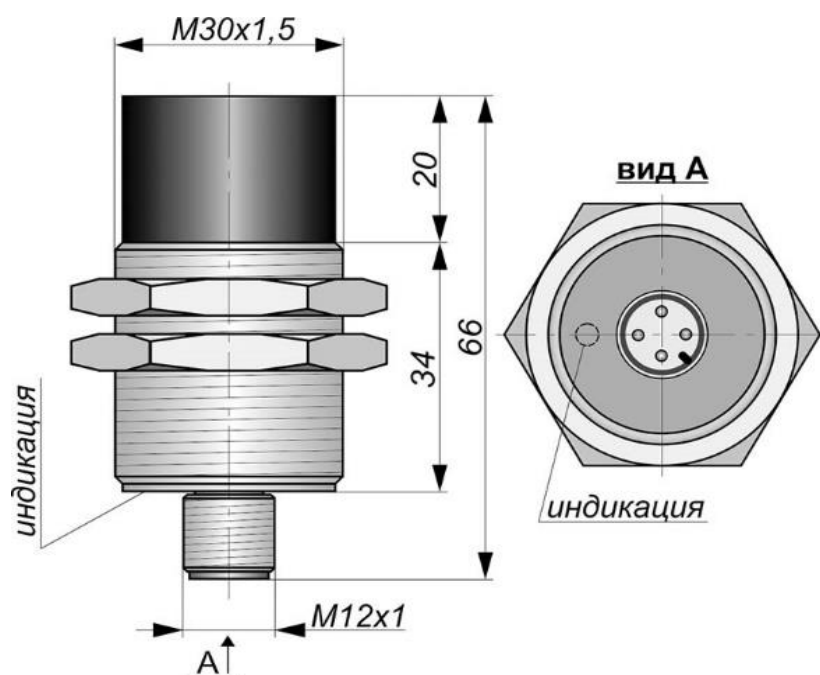
Габаритный чертеж
