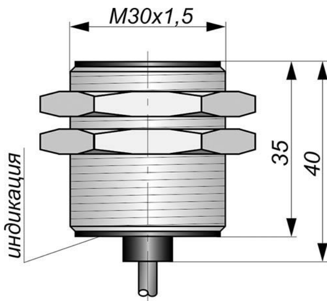
Габаритный чертеж
