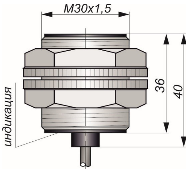
Габаритный чертеж
