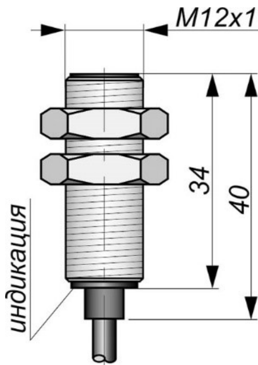
Габаритный чертеж
