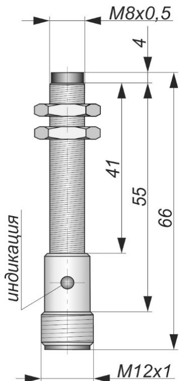
Габаритный чертеж
