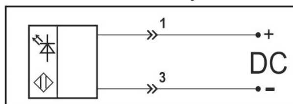
оптического излучателя
