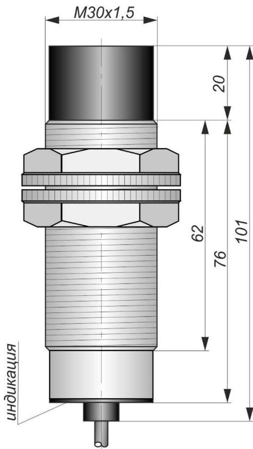
Габаритный чертеж
