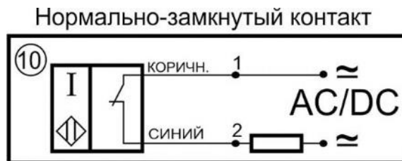
Схема соединения
