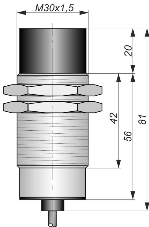
Габаритный чертеж
