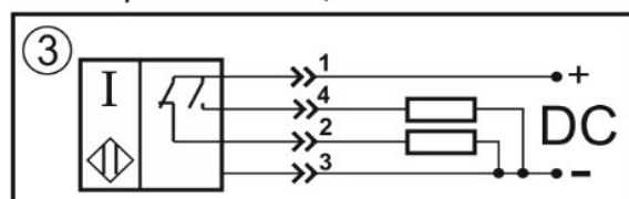
Переключающий контакт
