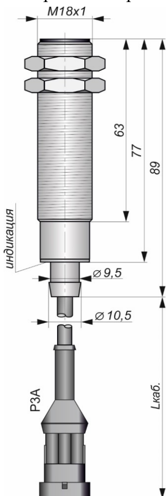
Габаритный чертеж
