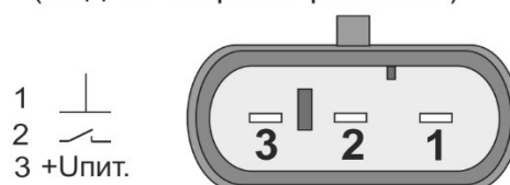
Нормально-разомкнутый контакт
