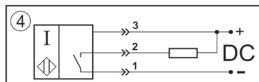
Нормально-разомкнутый контакт
