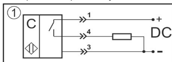
Нормально-разомкнутый контакт
