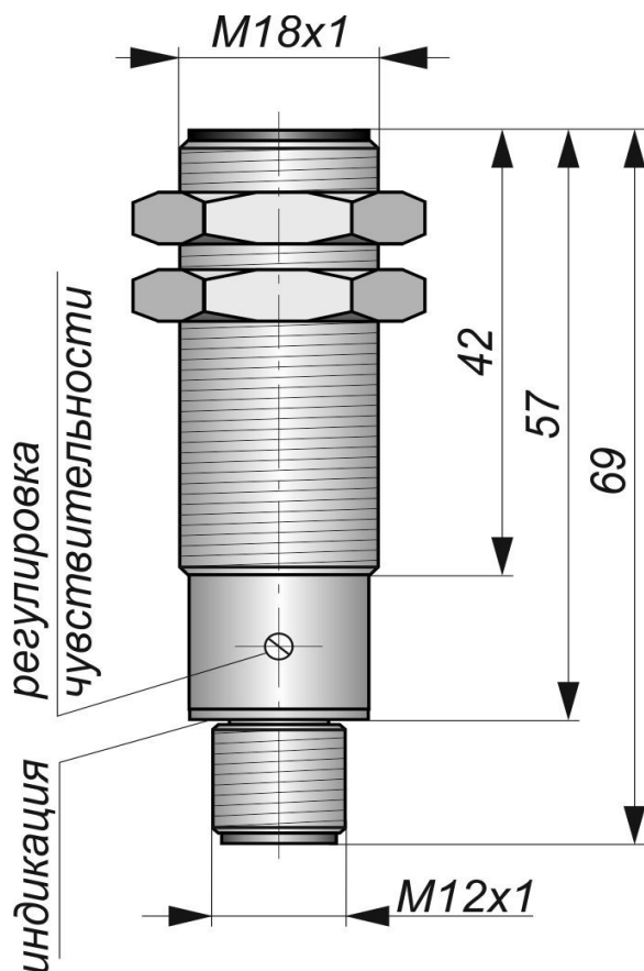
Габаритный чертеж
