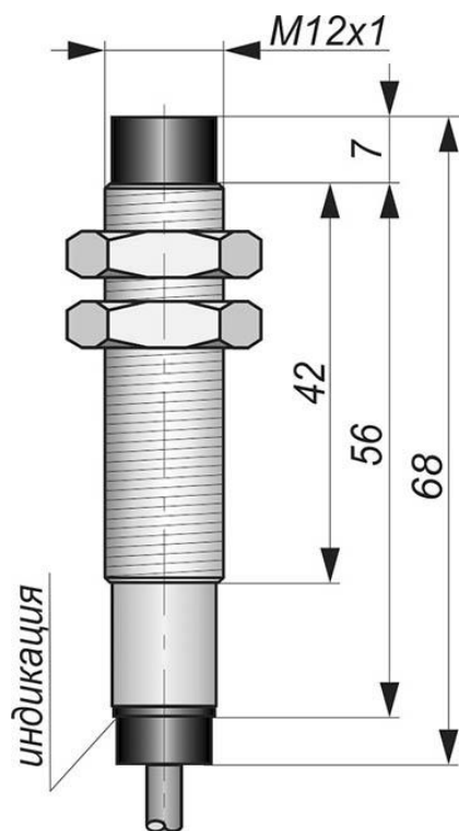
Габаритный чертеж
