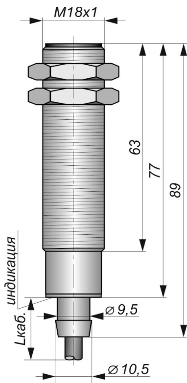
Габаритный чертеж
