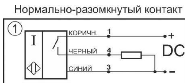
Схема соединения
