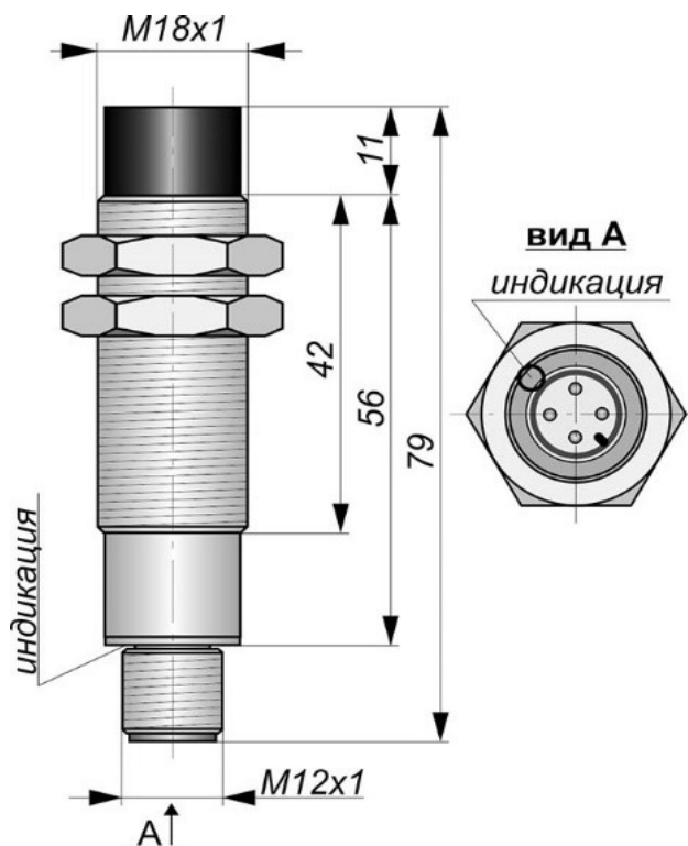
Габаритный чертеж
