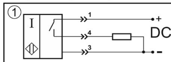
Нормально-разомкнутый контакт
