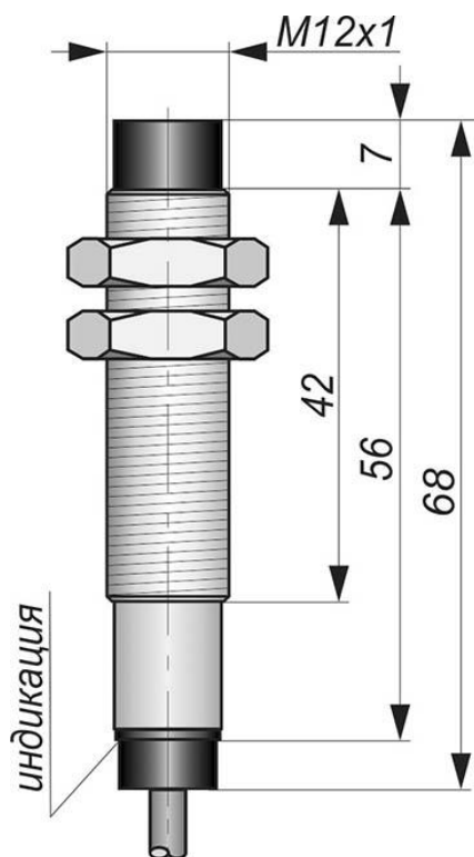
Габаритный чертеж
