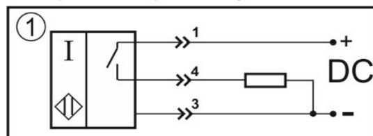
Цоколевка разъема
