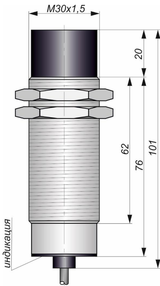
Габаритный чертеж
