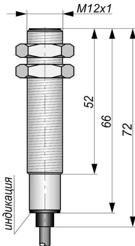
Габаритный чертеж
