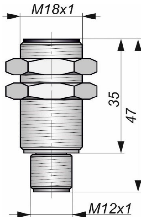
Габаритный чертеж
