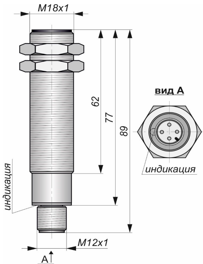
Габаритный чертеж
