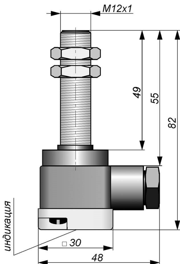
Габаритный чертеж
