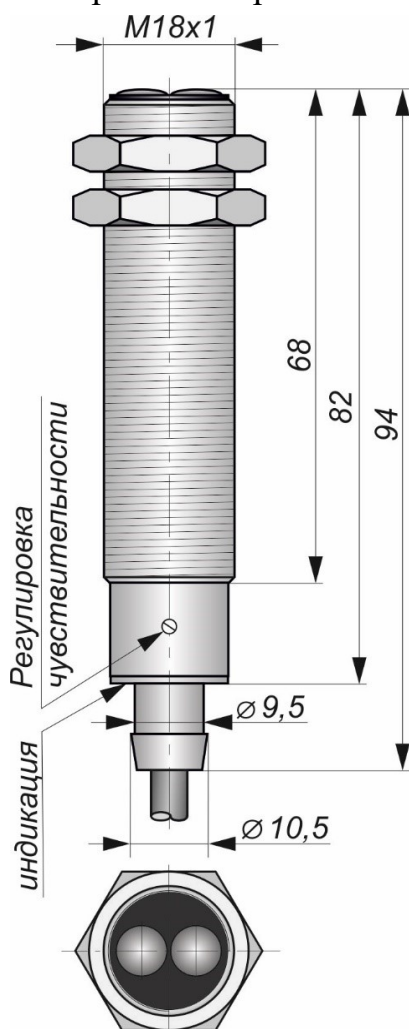
Габаритный чертеж
