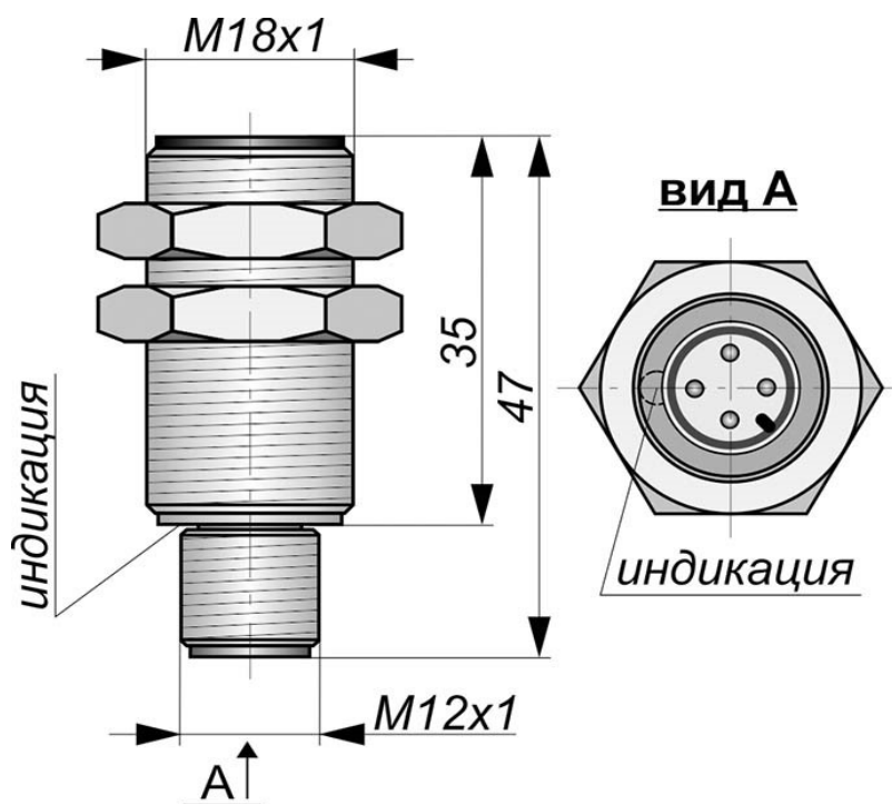
Габаритный чертеж
