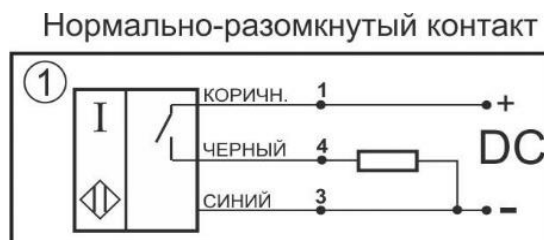
Схема соединения
