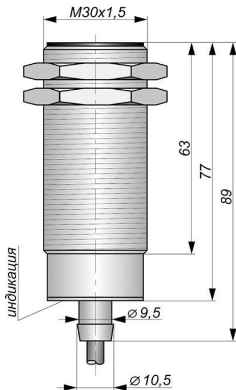
Габаритный чертеж
