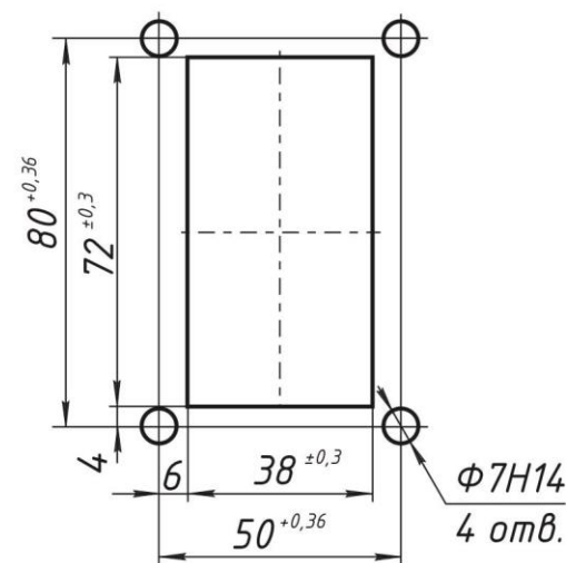
Посадочное место
