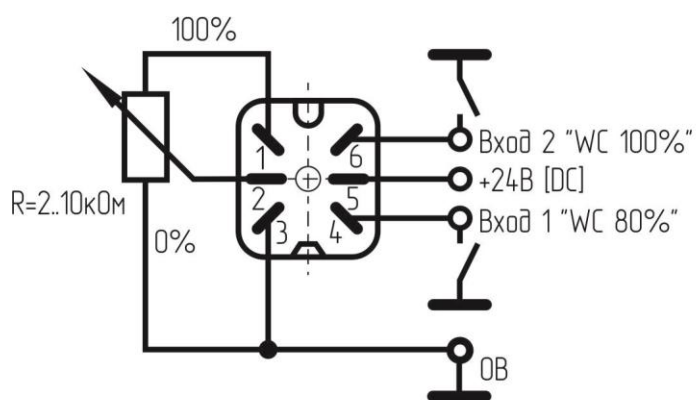
Схема подключения
