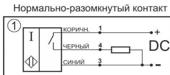
Схема соединения
