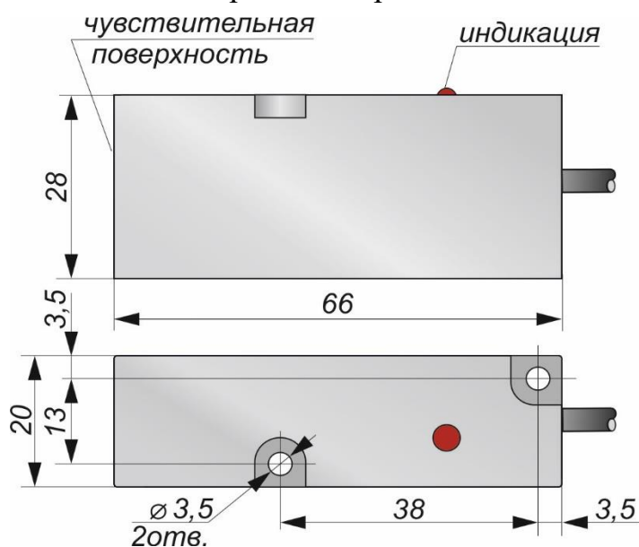
Габаритный чертеж
