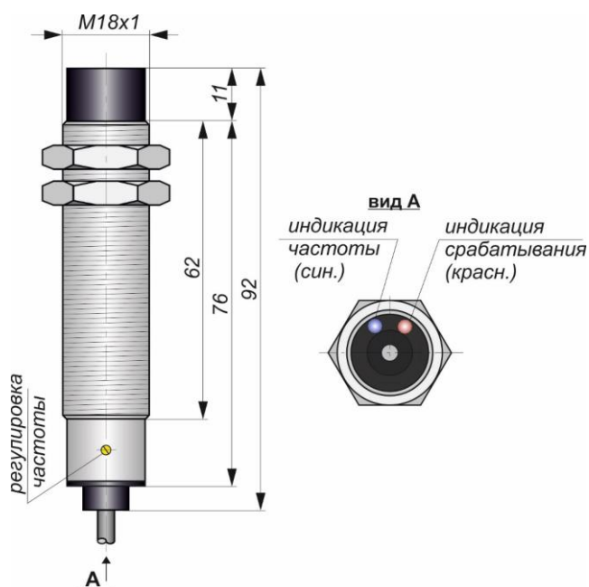
Габаритный чертеж
