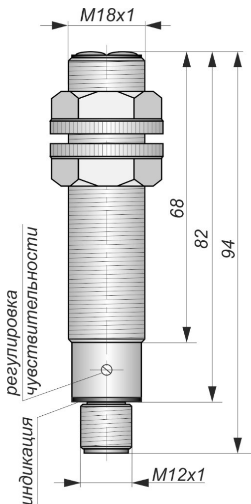
Габаритный чертеж
