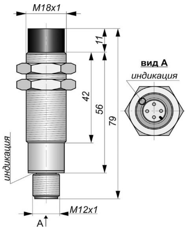
Габаритный чертеж
