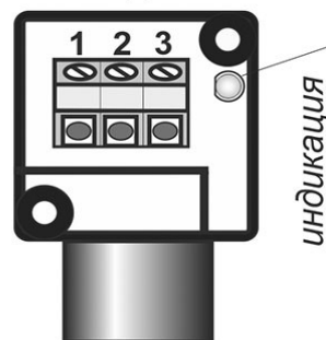
Цоколевка клеммной колонки
