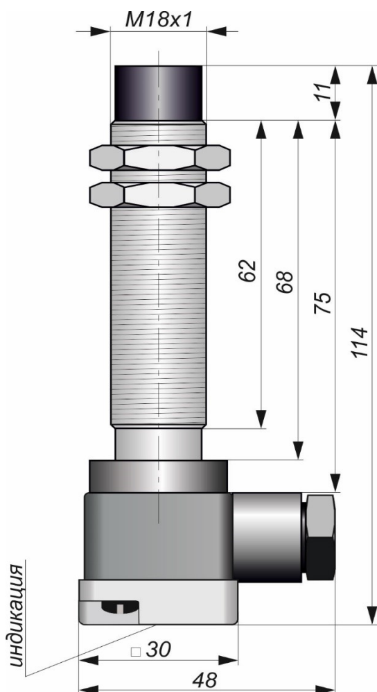
Габаритный чертеж
