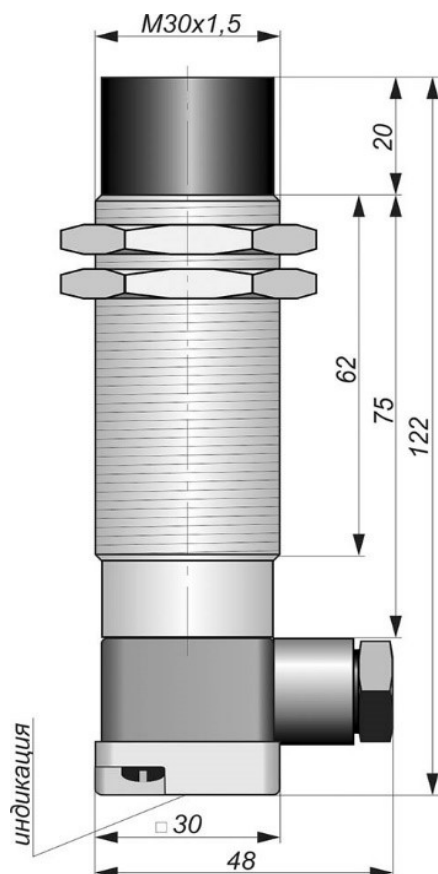
Габаритный чертеж
