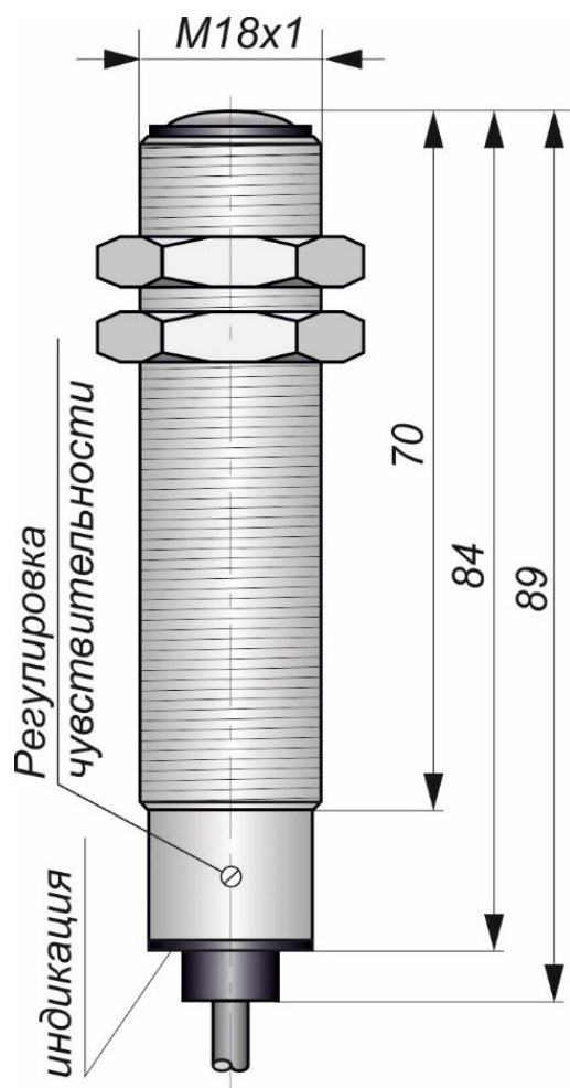
Габаритный чертеж
