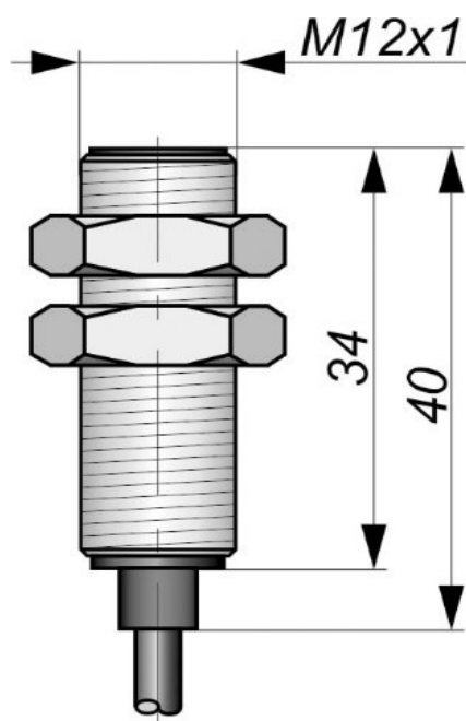
Габаритный чертеж
