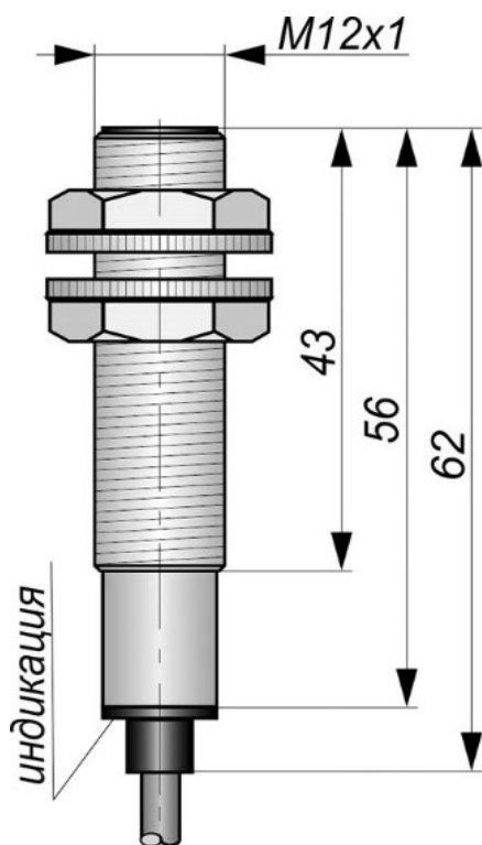
Габаритный чертеж
