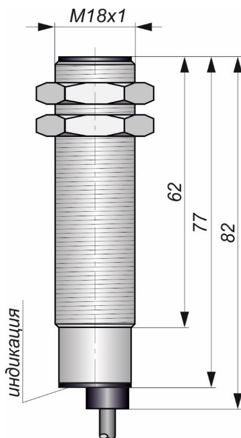
Габаритный чертеж
